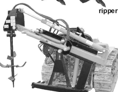
trivella idraulica
