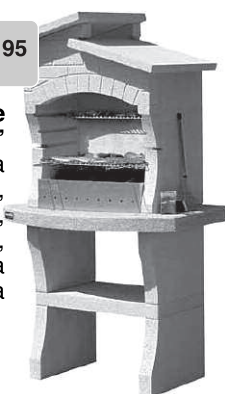
Barbecue "Assuan" in pietra ricostruita, cm 98x65xh176, griglia 60x40, a carbonella e legna
